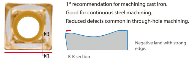
Tough edge GH chipbreaker
