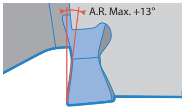
Dynamische Schneidkantenausführung
